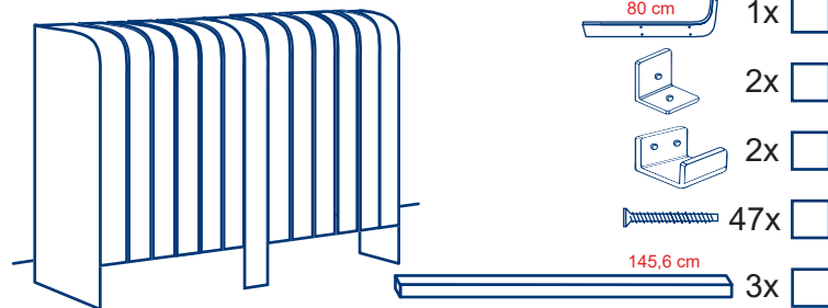
15 Holzleisten Modul Innenmaß 168,0 cm
